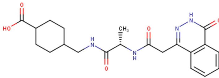
Gambar 1. Struktur molekul STK630921
