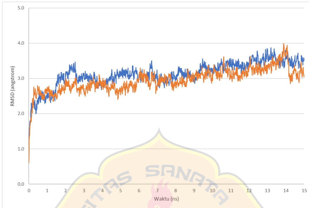
Gambar 2. Grafik nilai RMSD terhadap waktu selama simulasi. Kurva berwarna biru menunjukkan nilai RMSD pada simulasi dengan ligan dan kurva berwarna kuning menunjukkan nilai RMSD pada simulasi tanpa adanya ligan.
