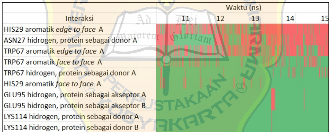
Gambar 4. Heatmap interaksi non hidrofobik pada interval simulasi 10 ns sampai 15 ns. Warna merah menunjukkan adanya interaksi, warna hijau menunjukkan tidak adanya interaksi. Huruf B menunjukkan molekul dimer B
