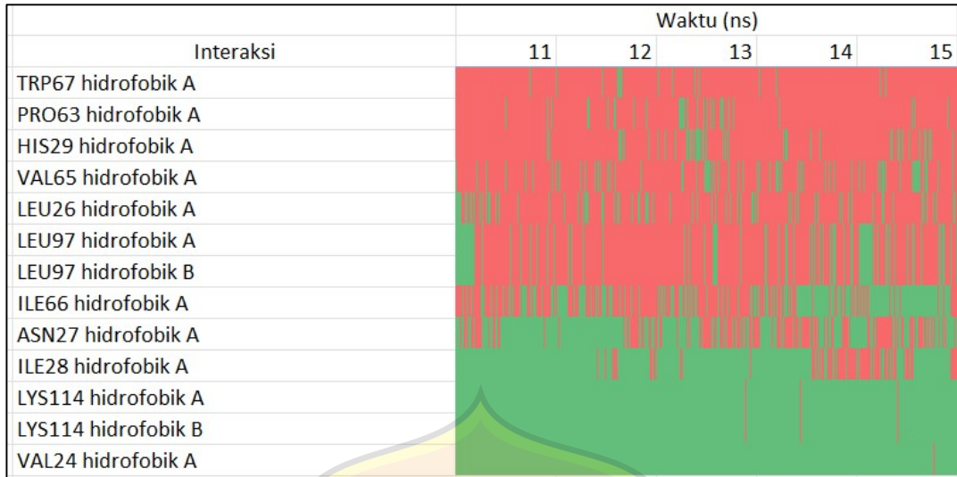
Gambar 3. Heatmap interaksi hidrofobik pada interval simulasi 10 ns sampai 15 ns. Warna merah menunjukkan adanya interaksi, warna hijau menunjukkan tidak adanya interaksi. Huruf A dan B masing-masing menunjukkan molekul dimer A dan B.
